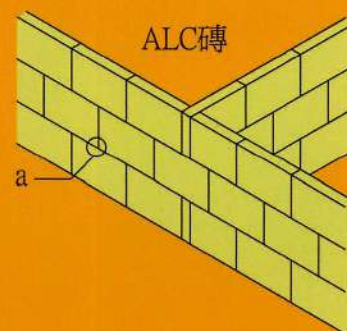
(L) 垂直交丁砌作
