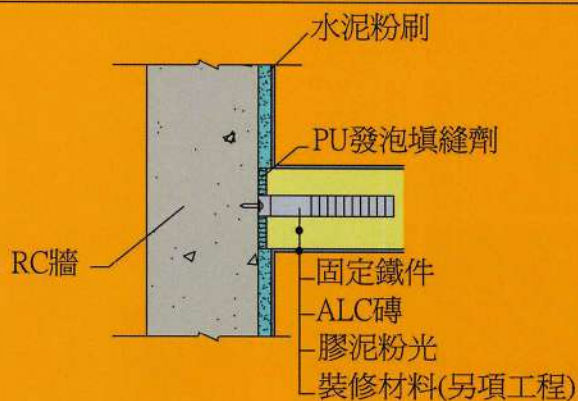
(B) ALC磚與RC牆剖面圖
