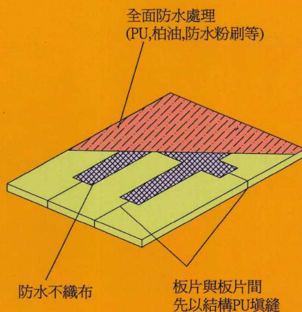
①R 防水處理
