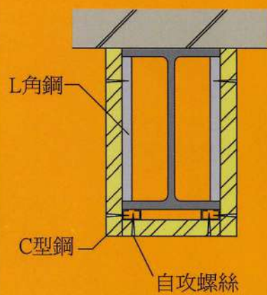
② 包覆樑
