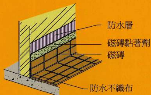
(M3) 防水處理
