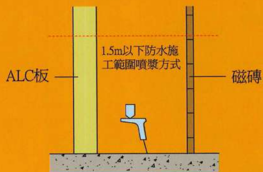
薄膜防水施工方法
