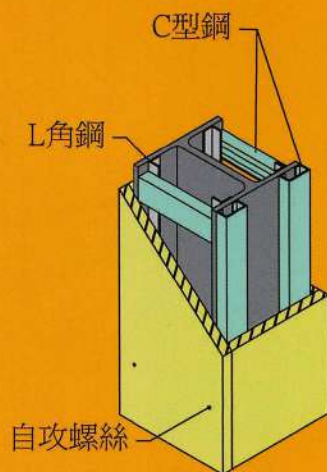
③ 包覆柱
