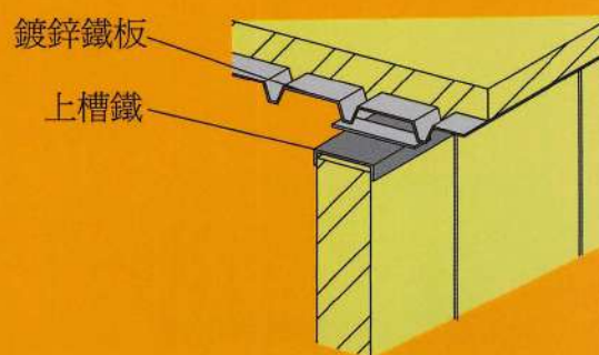
① F2 樓板交接
