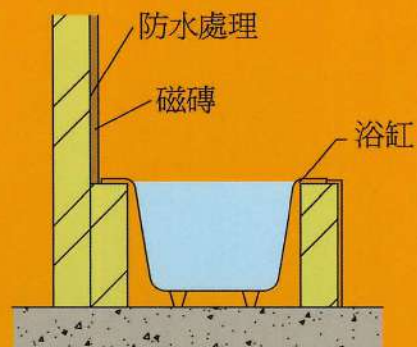
(M4) 浴缸池
