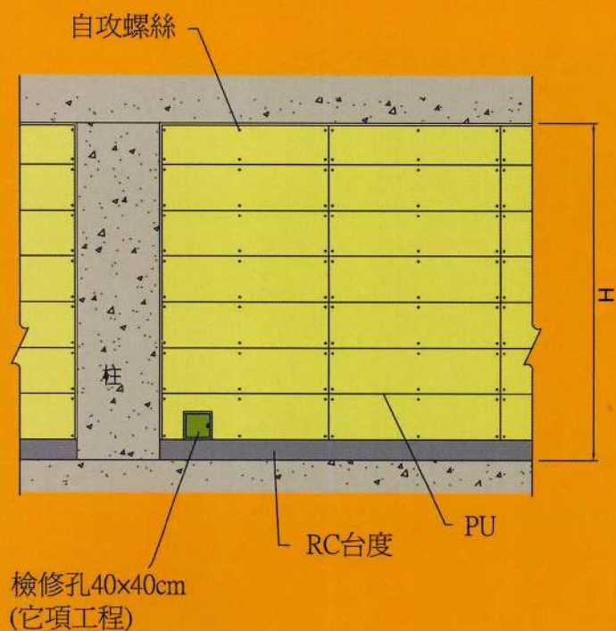
(S2) 地下室複壁-橫板工法
