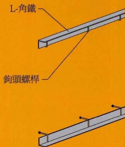
可拆解式工法
