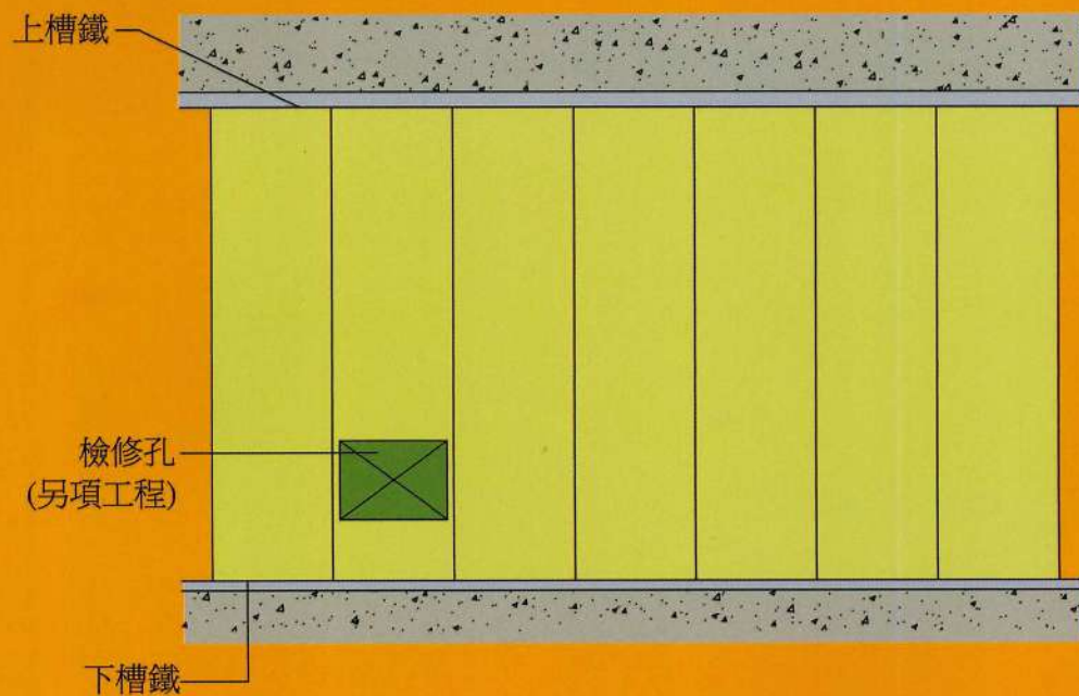
① 地下室複壁-直板工法
