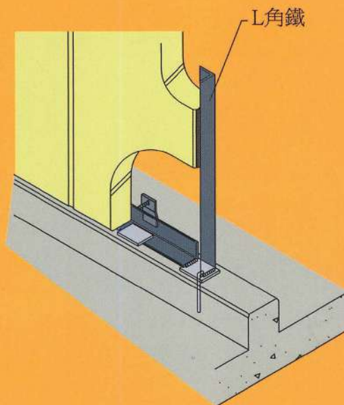
①k 陽台落地門
