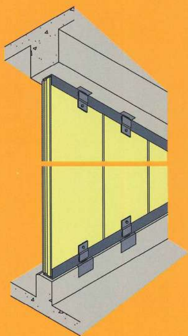
①h2 退縮陽台牆
