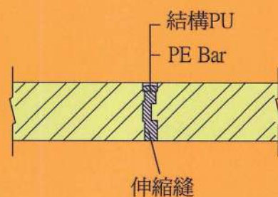
A-A剖面詳圖
