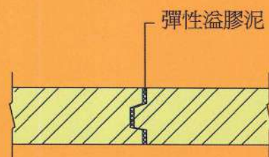
B-B剖面詳圖
