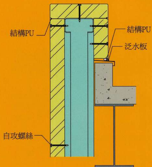
② 女兒牆 (ALC蓋板)
