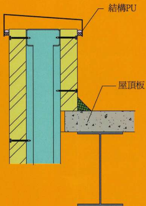
① 女兒牆 (金屬蓋板)
