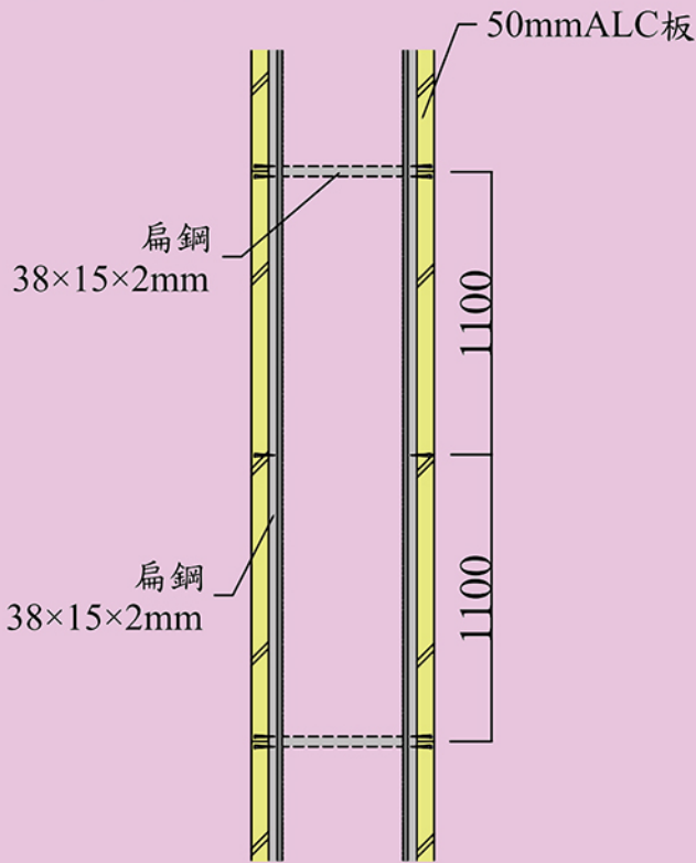
垂直斷面圖
